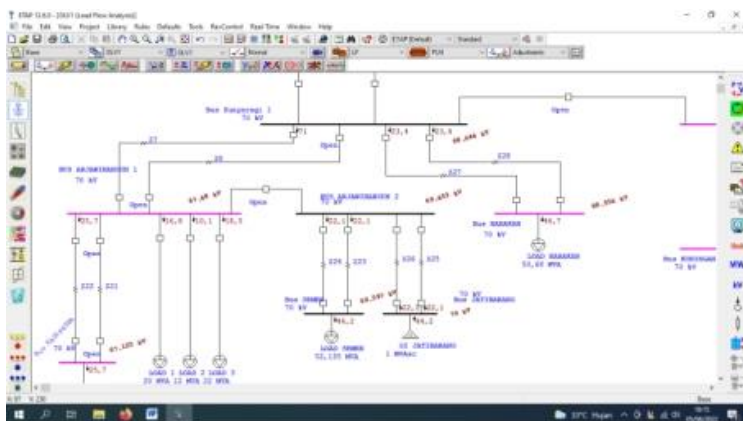
Gambar 12, Tegangan bus 2 Arjawinangun sebelum PMT Jtbrg 1 gangguan
