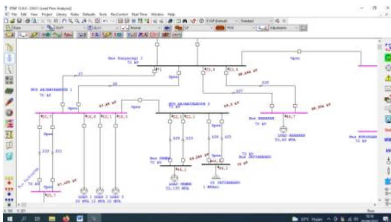
Gambar 13, Tegangan bus 2 Arjawinangun PMT Jtbrg 1 terjadi gangguan
