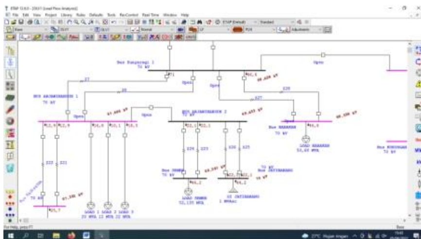
Gambar 9, Tegangan bus 1 Sunyaragi PMT BBKAN 1 terjadi gangguan
