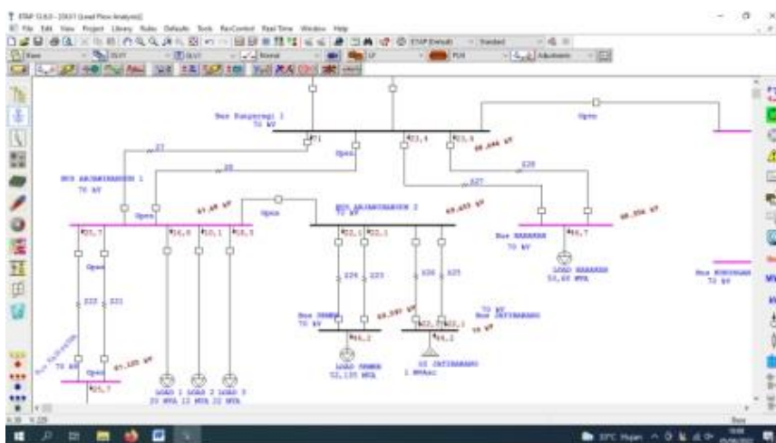
Gambar 11, Tegangan bus 1 Arjawinangun PMT Kdptn terjadi gangguan
