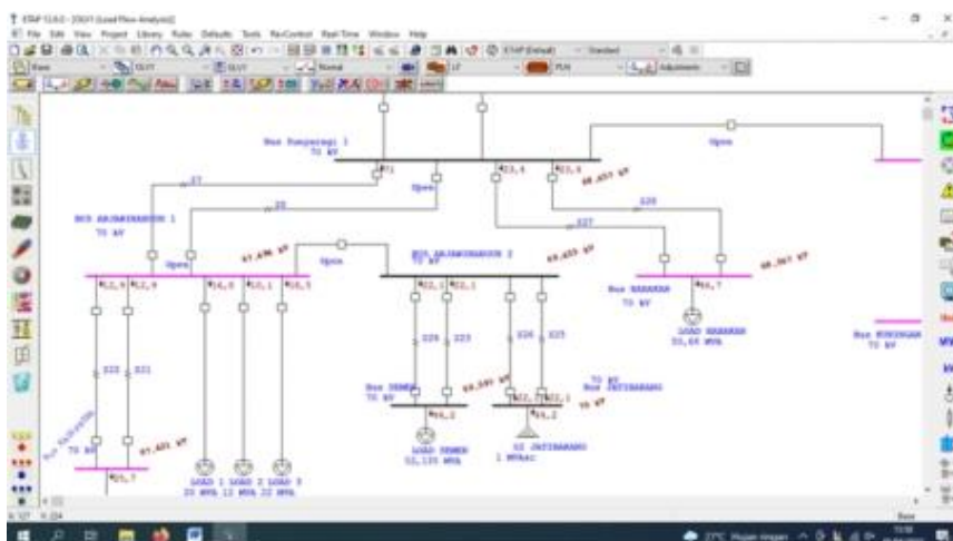
Gambar 8, Tegangan bus 1 Sunyaragi sebelum PMT BBKN 1 gangguan
