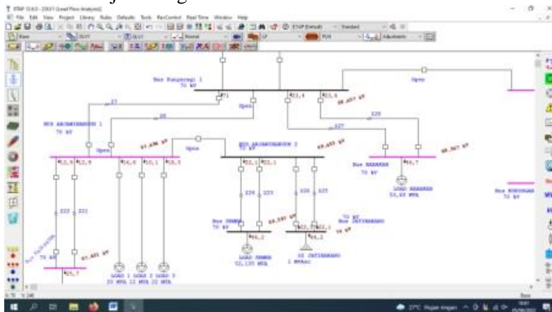
Gambar 10, Tegangan bus 1 Arjawinangun sebelum PMT Kdptn gangguan
